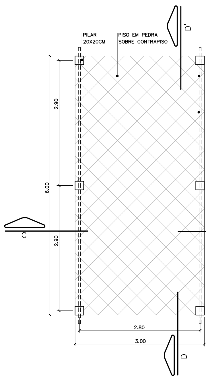
PLANTA DE PISO DO PERGOLADO ESC. 1:50
