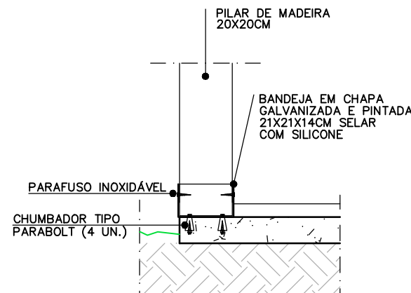
DET. 02 BASE PILAR ESC. 1:20
