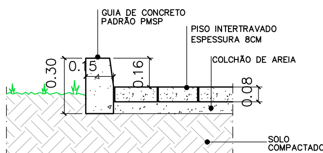
DET. GUIA DE CONCRETO ESC. 1:20
