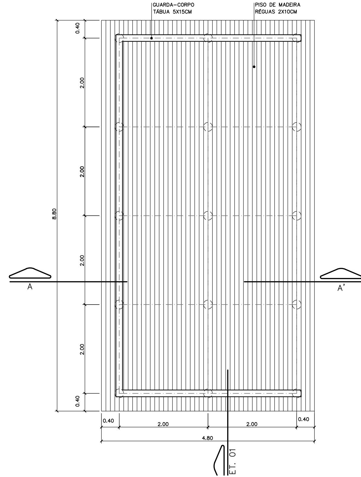
ESTRUTURA DO DECK ESC. 1:50
