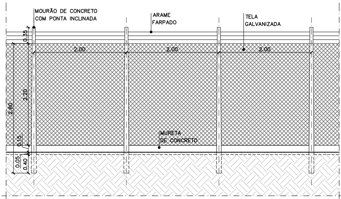
VISTA FECHAMENTO ESC. 1:50
