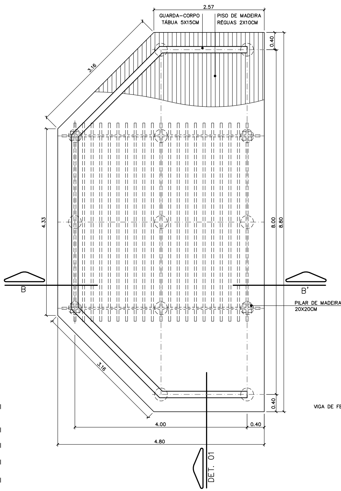
PLANTA DO MIRANTE ESC. 1:50
