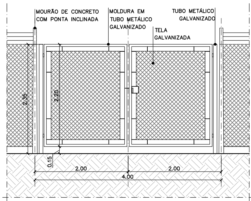
VISTA PORTÃO ESC. 1:50
