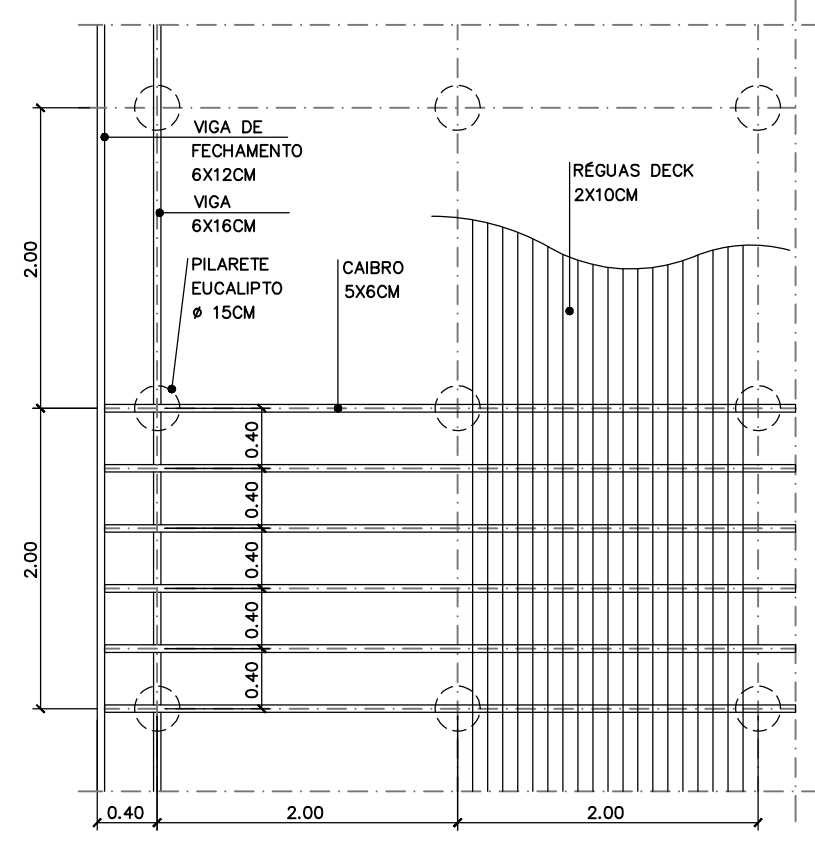
ESTRUTURA DO DECK ESC. 1:50
