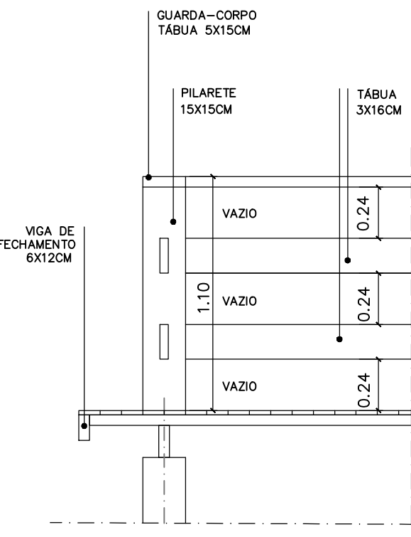
DET. 01 GUARDA-CORPO ESC. 1:25
