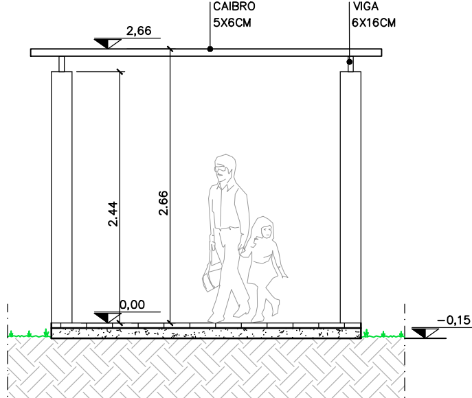
CORTE C - C' ESC. 1:50
