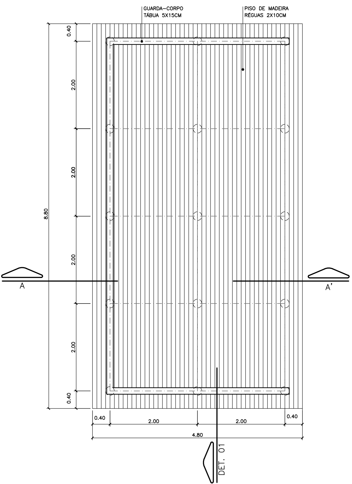
PLANTA DO DECK ESC. 1:50
