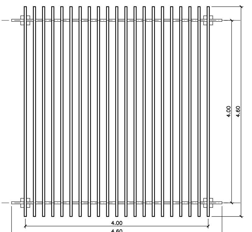
PLANTA DO PERGOLADO DO MIRANTE ESC. 1:50
