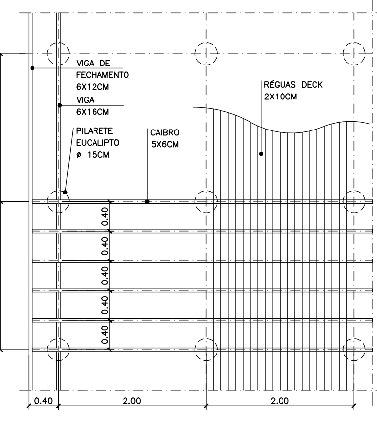
ESTRUTURA DO DECK ESC. 1:50
