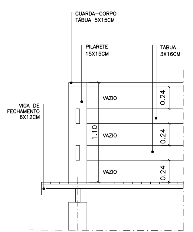
DET. 01 GUARDA-CORPO ESC. 1:25
