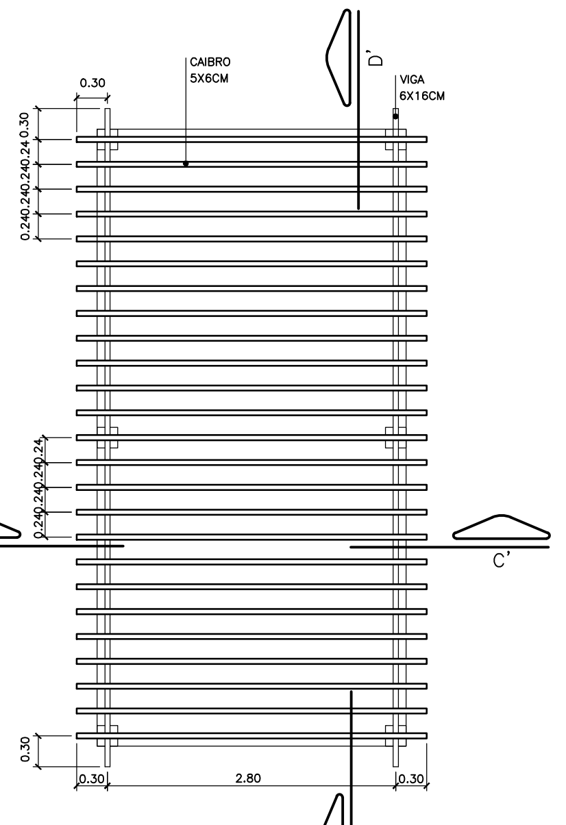
PLANTA DO PERGOLADO ESC. 1:50
