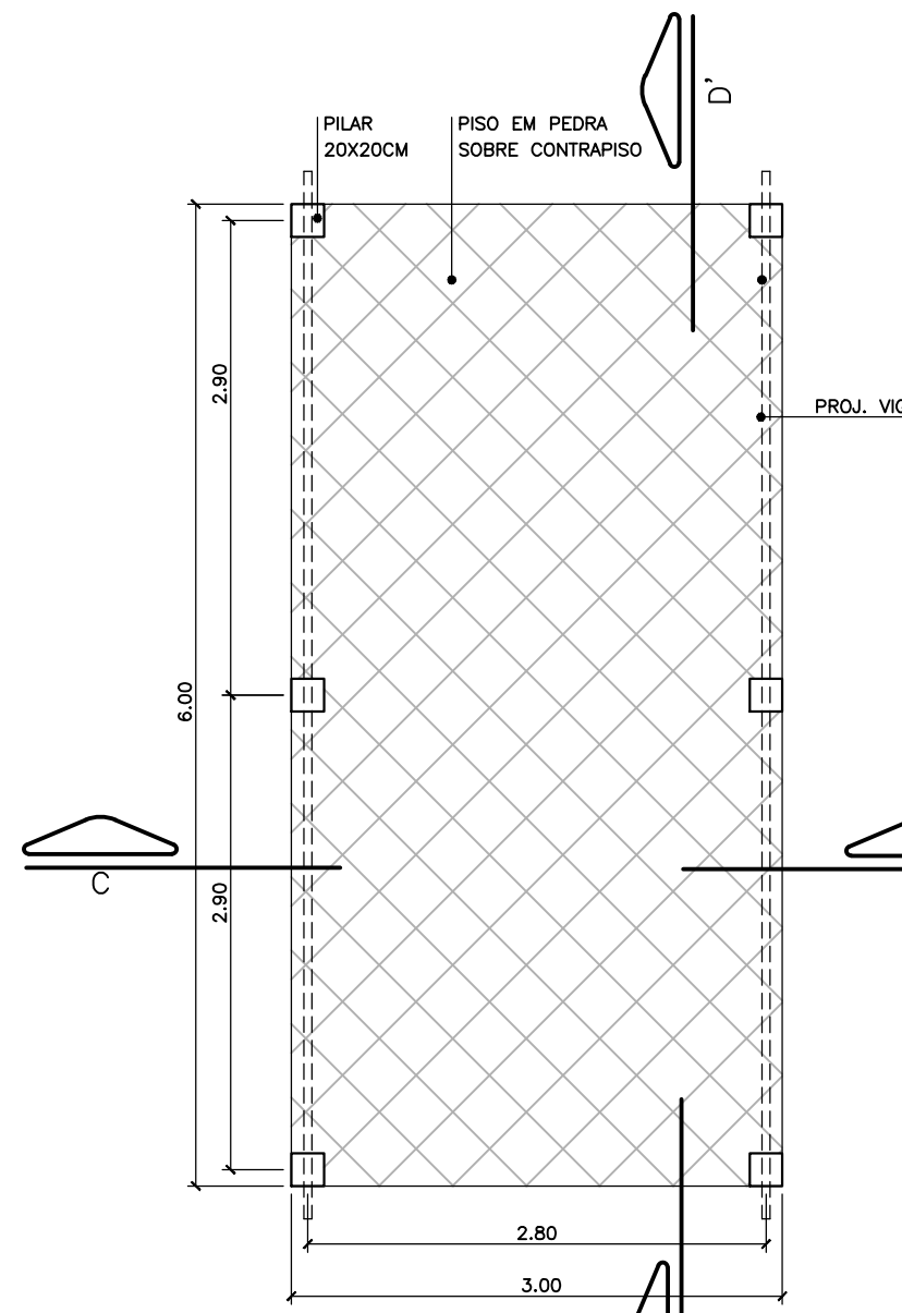
PLANTA DE PISO DO PERGOLADO ESC. 1:50
