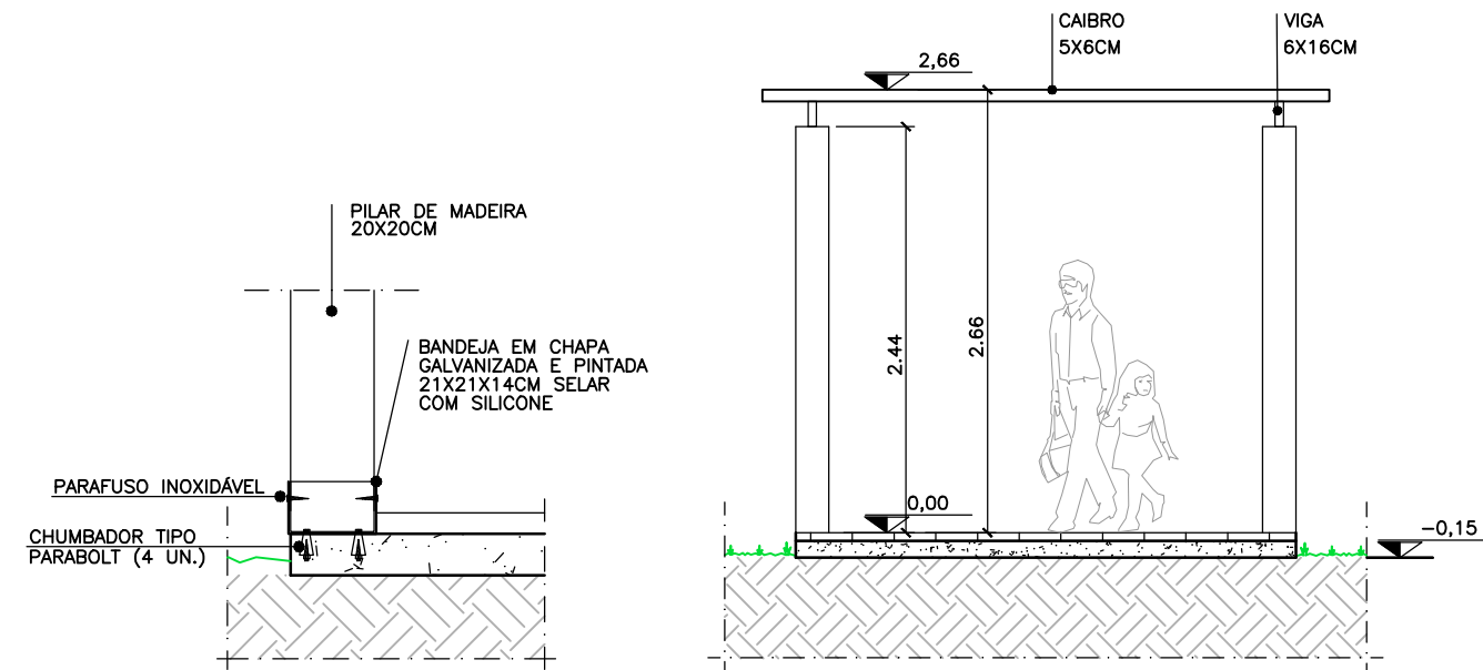
DET. 02 BASE PILAR ESC. 1:20
