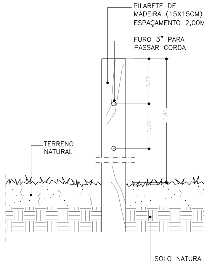
DETALHE 03 ESC. 1:10
