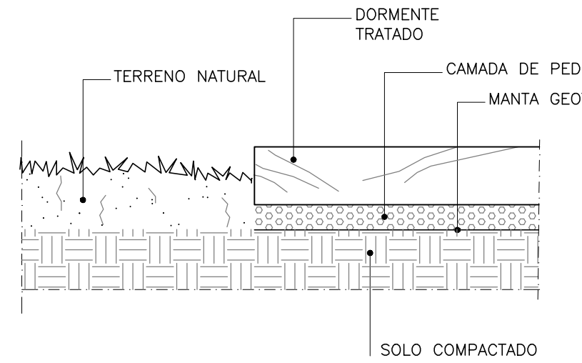
DETALHE 02 ESC. 1:10
