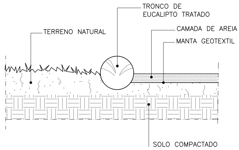
DETALHE 01 ESC. 1:10
